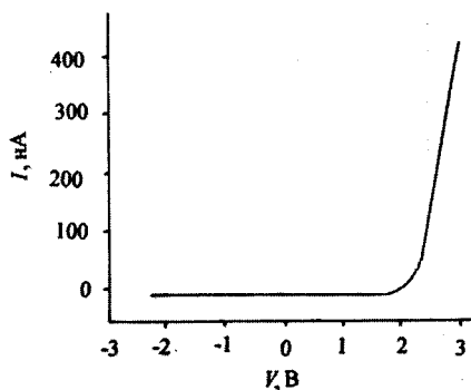
Рис.4. Выпрямляющий диод на изогнутой нанотрубке. Нанотрубка лежит на непроводящей (кварцевой) подложке в контакте с двумя сверхтонкими проводниками (а); вольт-амперная характеристика для такой системы (б).
