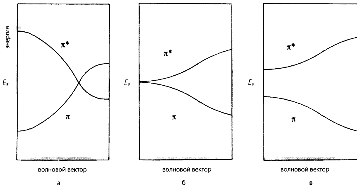
Рис.2. Электронная структура нехиральных трубок: а) все трубки (n, n) металлические; трубки (n, 0) металлические, если n кратно трем (б), иначе они полупроводниковые (в). Уровень Ферми E_F разделяет занятые и вакантные состояния.
