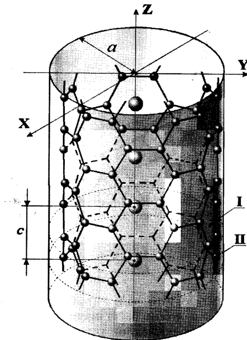
Рис.8. Легированная металлом (цветные шарики) углеродная нанотрубка внутри цилиндрического потенциального барьера. I — область постоянного межатомного потенциала, II — область атомного потенциала. (При расчетах атомные сферы считаются касающимися друг друга.)
