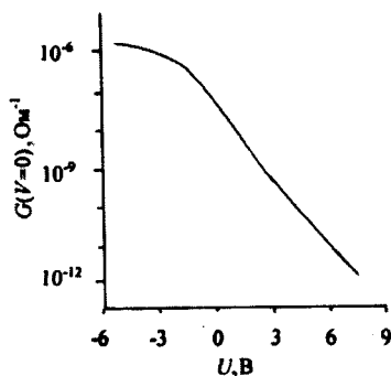
Рис.5. Полевой транзистор на полупроводниковой нанотрубке. Нанотрубка лежит на непроводящей (кварцевой) подложке в контакте с двумя сверхтонкими проводниками, в качестве третьего электрода (затвора) используется кремниевый слой (а); зависимость проводимости в цепи от потенциала затвора (б).
