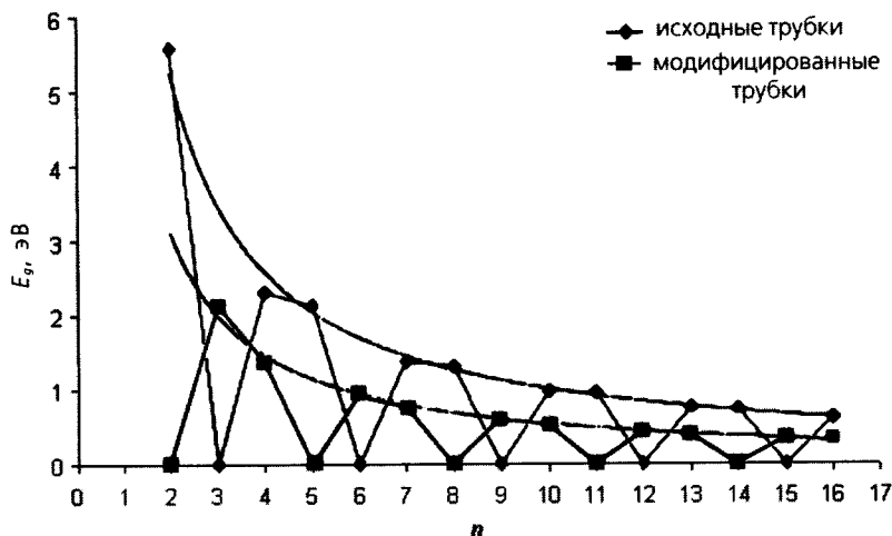
Рис.9. Зависимость ширины запрещенной зоны для исходных и модифицированных нанотрубок типа (n, 0) от параметра их диаметра n .
