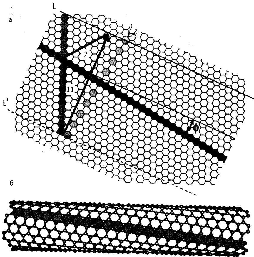
Рис.1. Построение модели нанотрубки: а) графитовый слой и лента (11, 7); б) нанотрубка (11, 7). Кроме индексов (n, m) , геометрию нанотрубки можно охарактеризовать длиной окружности цилиндра C и углом хиральности \Phi . Если вектор C совпадает с вертикальной или наклонной «разрезанной» линией шестиугольников, получаются нехиральные трубки (n, 0) и (n, n) .
