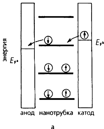
Рис.6. Схема переноса электронов с участием одного дискретного уровня в полевом транзисторе на металлической нанотрубке (а) и зависимость проводимости в цепи от потенциала затвора (б).
